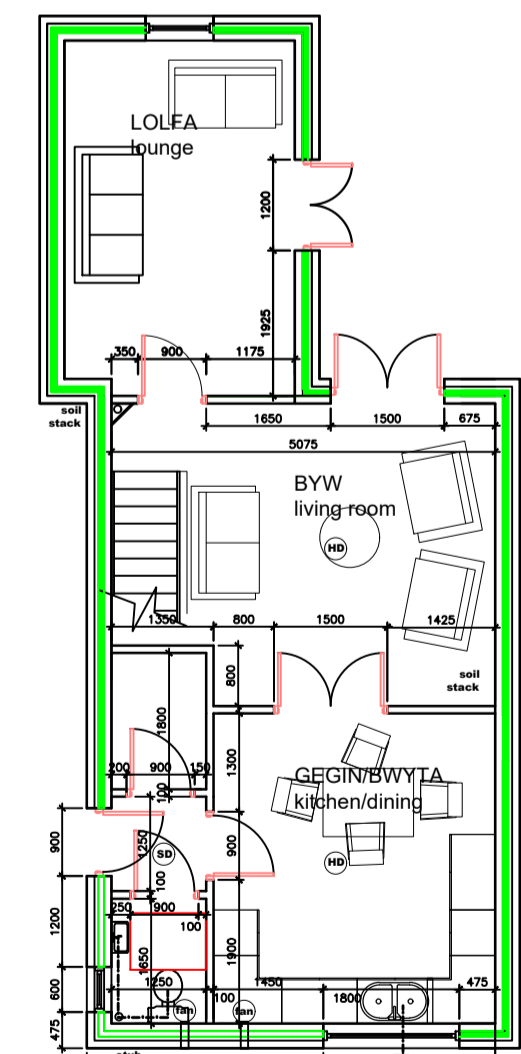
CYNLLUN Y LLAWR GWAELOD ground floor plan
