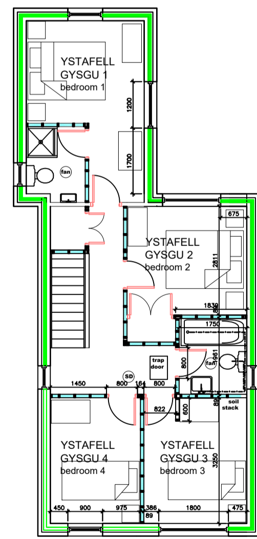
CYNLLUN Y LLAWR CYNTAF first floor plan
