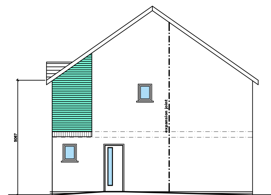
EDRYCHIAD OCHR side elevation
