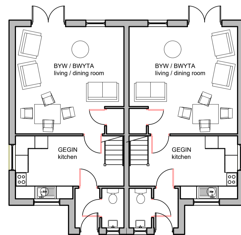
CYNLLUN Y LLAWR GWAELOD ground floor plan
