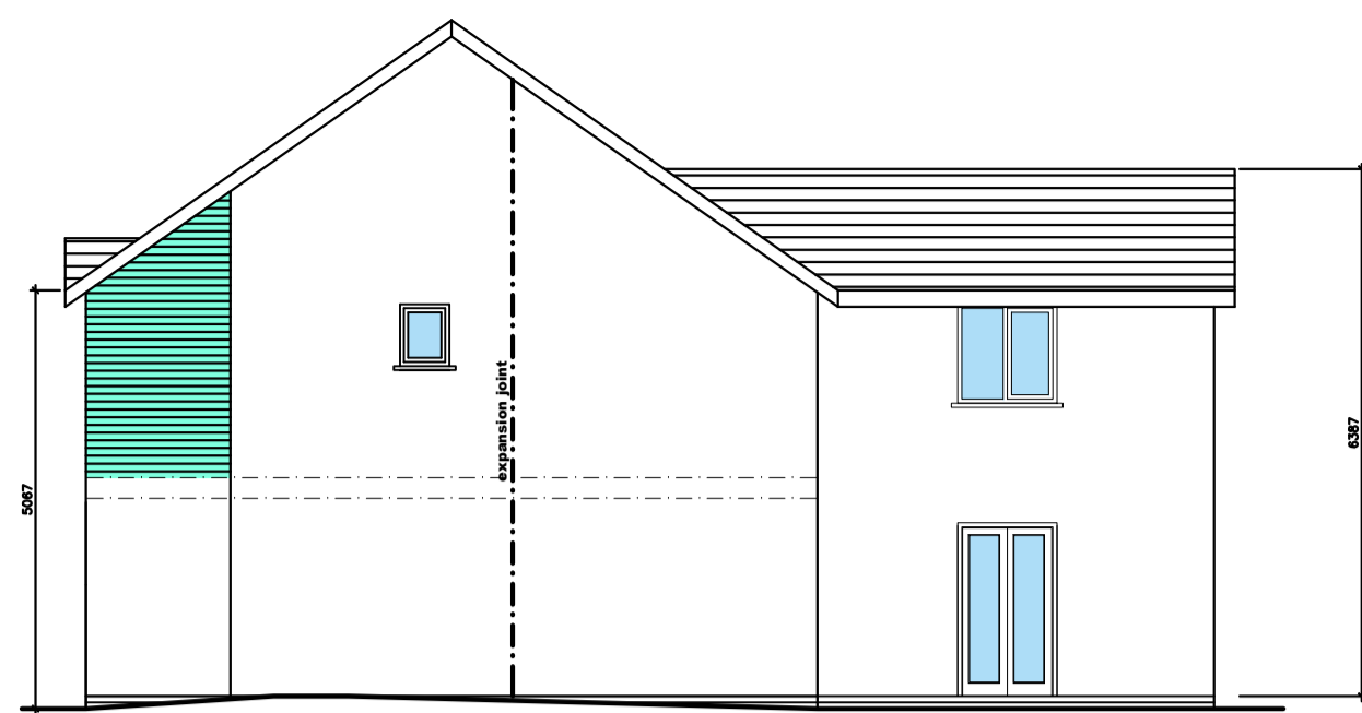
EDRYCHIAD OCHR side elevation
