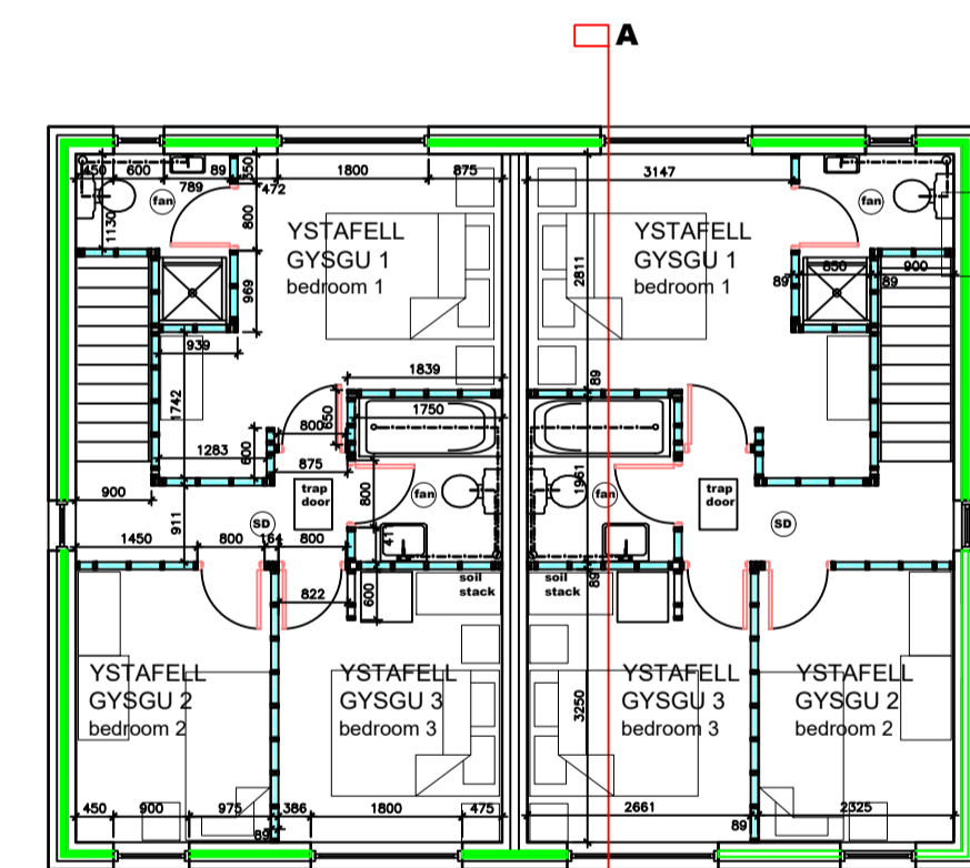
CYNLLUN Y LLAWR CYNTAF first floor plan
