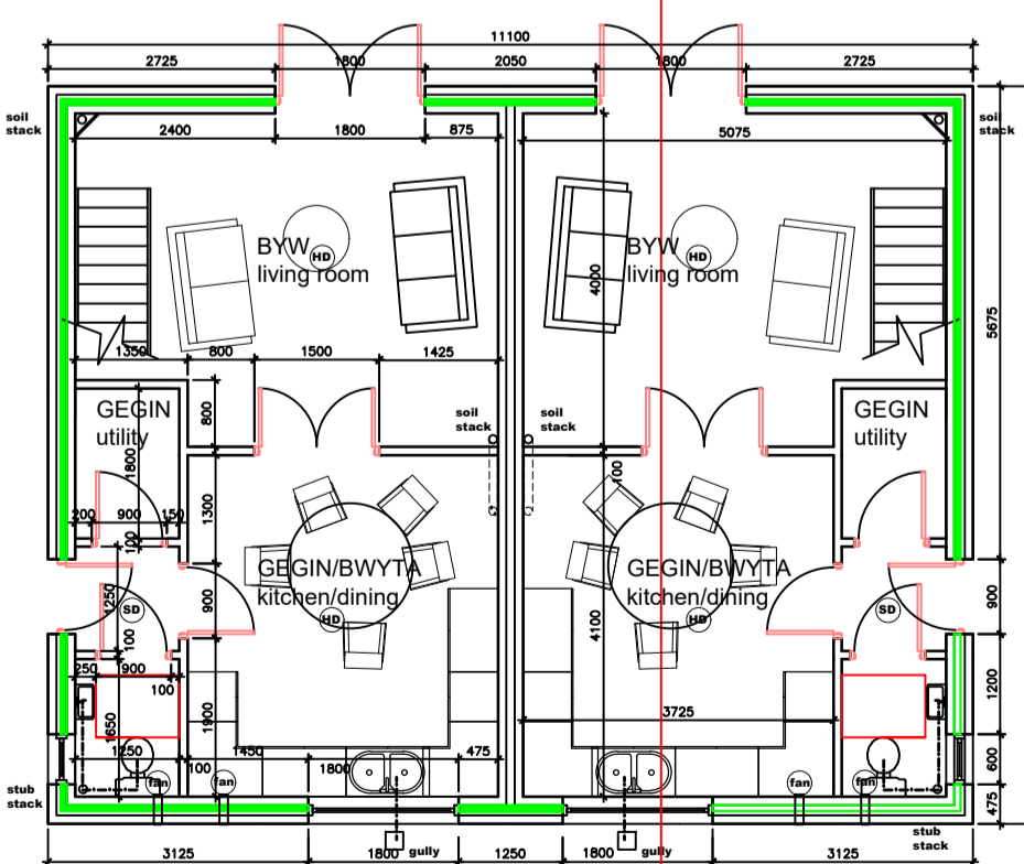
CYNLLUN Y LLAWR GWAELOD ground floor plan
